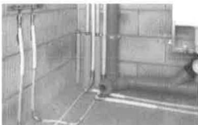
Beispiel REHAU HIS 311 Schiebehülse
